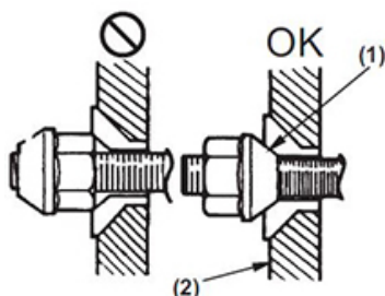
(1) Wheel Nut (2) Wheel Rim
